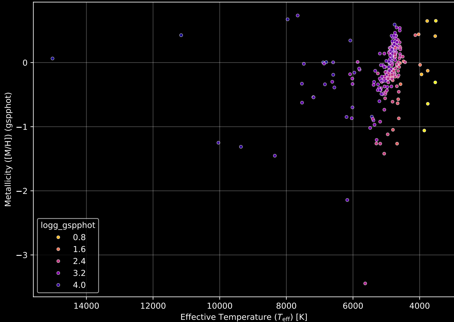
APOGEE DR17 Field: [010+04] Stellar Population Parameters (n= 259)
